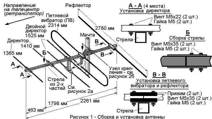
Рисунок 1 - Сборка и установка антенны
