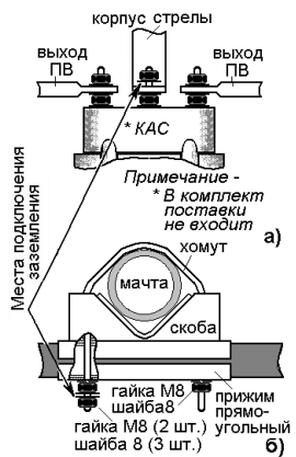
Рисунок 2 - Сборка узла крепления и заземление антенны
