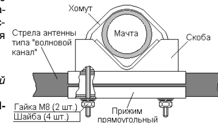
Рисунок 8 - Сборка узла крепления
