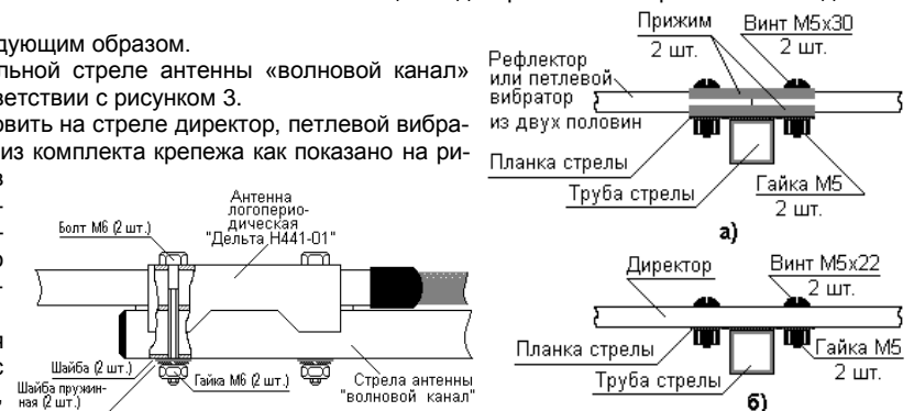
Рисунок 3 - Соединение антенн
