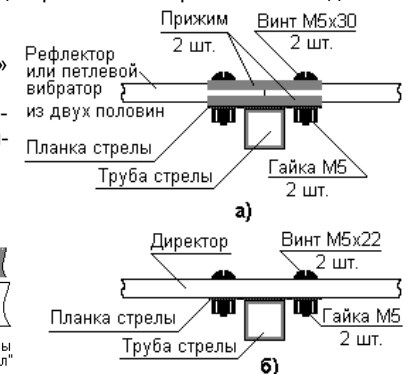
Рисунок 4 - Установка вибраторов
