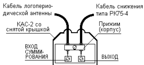
Рисунок 6 - Подключение кабелей к КАС
