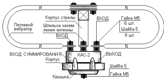
Рисунок 5 - Подключение КАС. Заземление антенны
